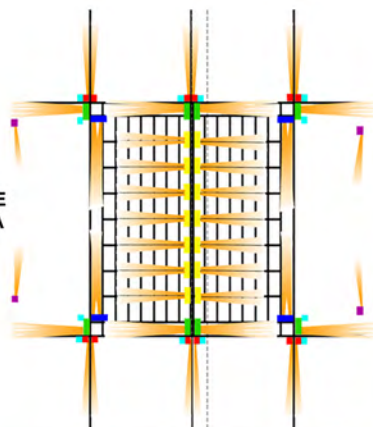
PLAN D'IMPLANTATION DE L'ECLAIRAGE LEDS DE LA GRANDE SALLE
